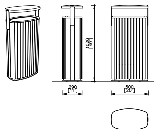
08 BIN 1:50 5002
